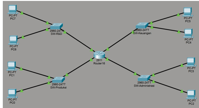
Gambar 1: Topologi menggunakan Cisco Packet Tracer
